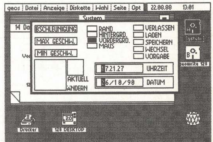
[2] Bildschirmfarben, Datum und Uhrzeit definiert das Hilfsprogramm »Voreinstellungen«
