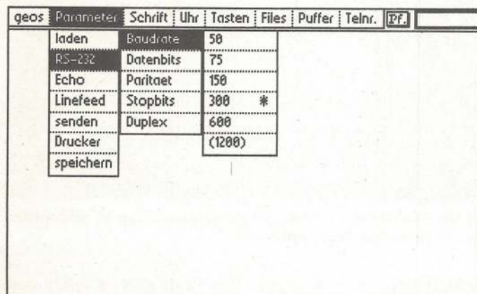
[6] Die Welt am Draht mit Geos: Geoterm bietet alle Funktionen professioneller DFÜ-Programme
