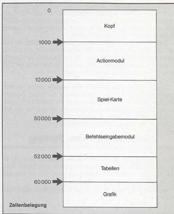
Bild 17. Sauber und übersichtlich: die ideale Programmaufteilung eines Basic-Adventures
