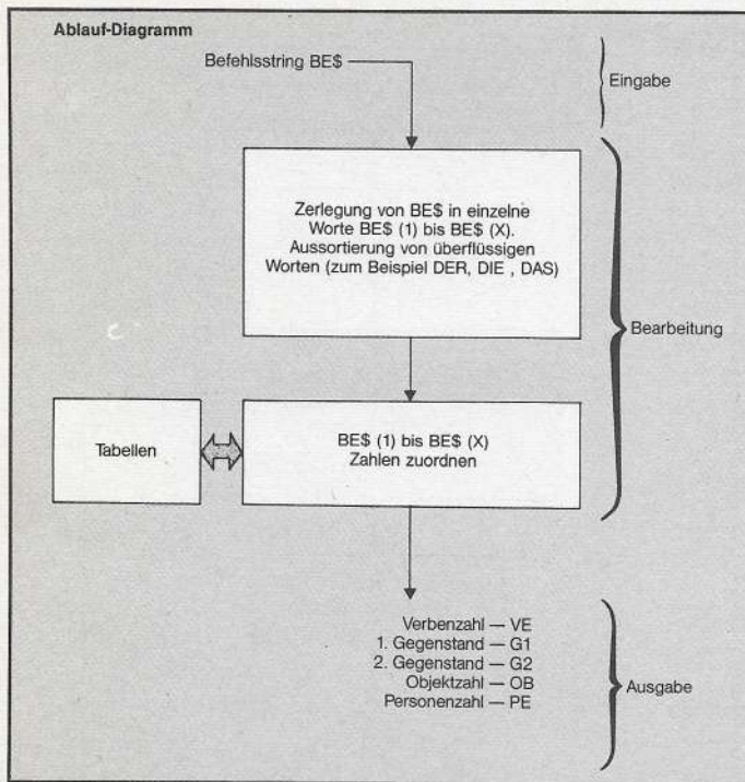
Bild 12. Funktionsweise des Codierungsmoduls
