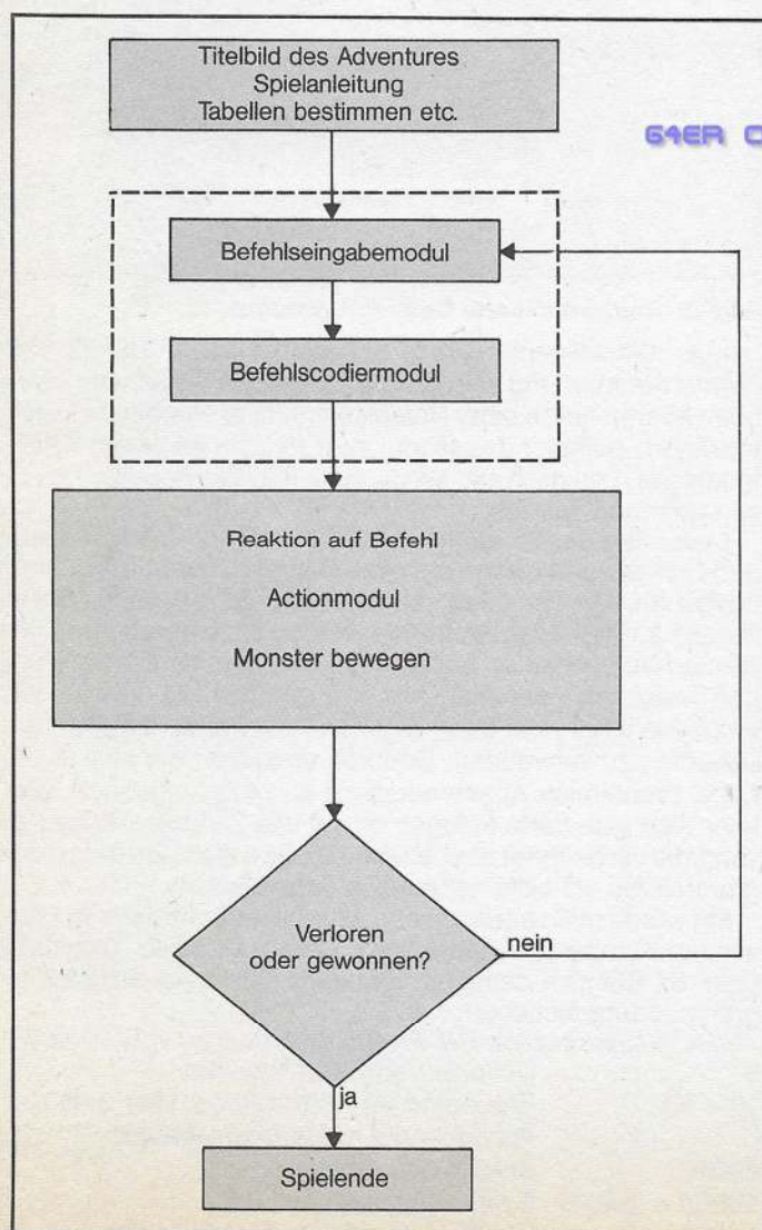
Bild 14. Der Ablaufplan unseres Adventures
