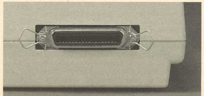
Bild 2. Die Centronics-Parallel-Schnittstelle
