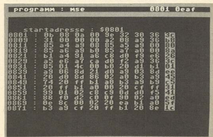
Das MSE-Programm dient der leichten und fehlerfreien Eingabe von Maschinensprache-Listings.
