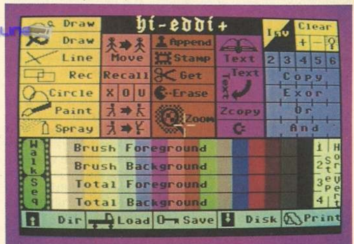
Bild 2. Das Menü von »Hi-Eddi«. Alle Funktionen können per Joystick angewählt werden
