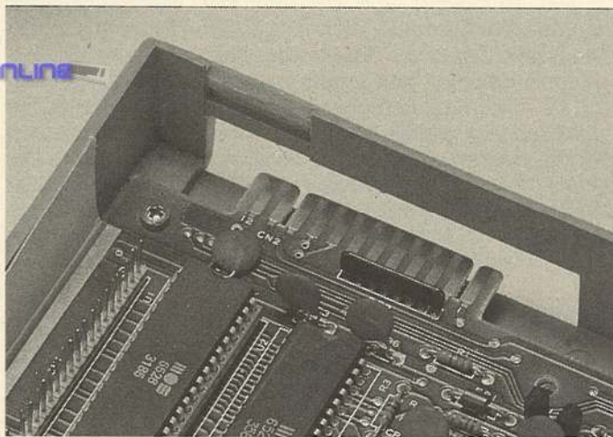
Bild 7. Der User-Port des C64
