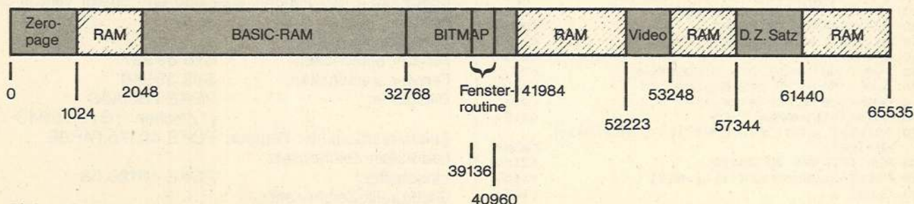
Bild 2. Die aktuelle Speicherbelegung
