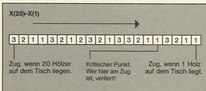
Bild 1. Strategie des Spielprogramms
