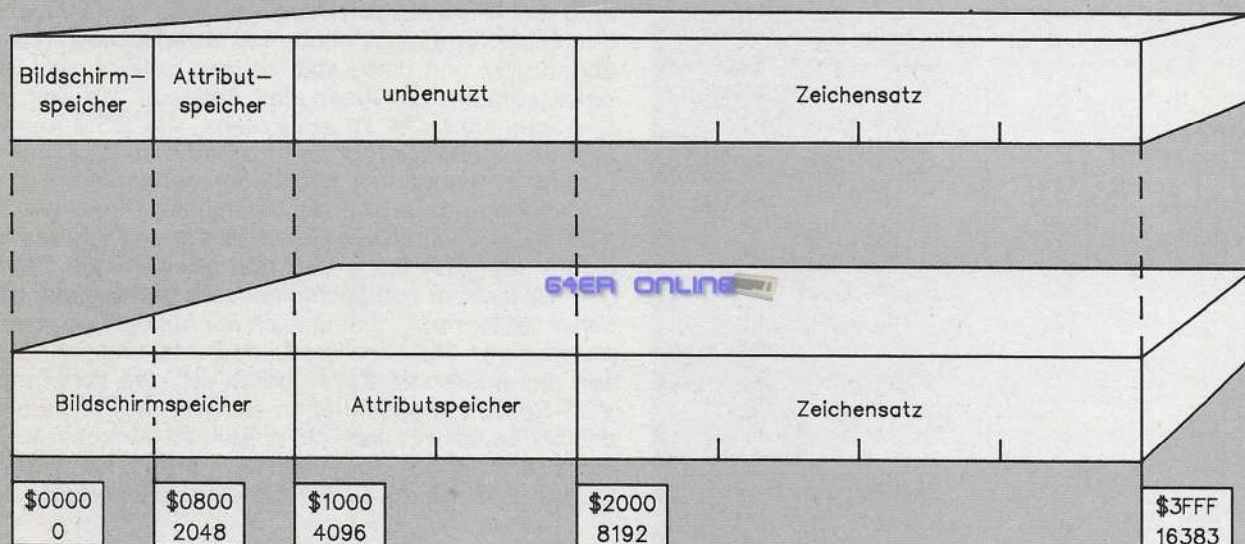
Bild 2. Die VDC-Speicherbelegung mit (unten) und ohne Interlace (oben). Einige Blöcke werden dabei verschoben.
