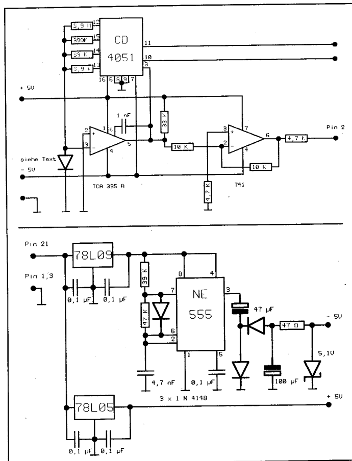
Luxmeter-Schaltplan: Spannungsversorgung und Meß-Schaltung
