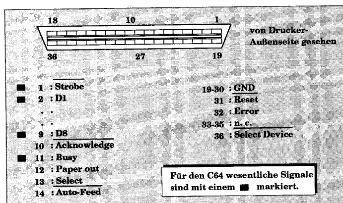
1 Belegung der Centronics-Schnittstelle
