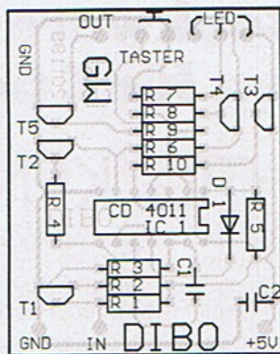
2 Bestückungsplan des elektronischen Diskettenlochers Verhältnis 1:1
