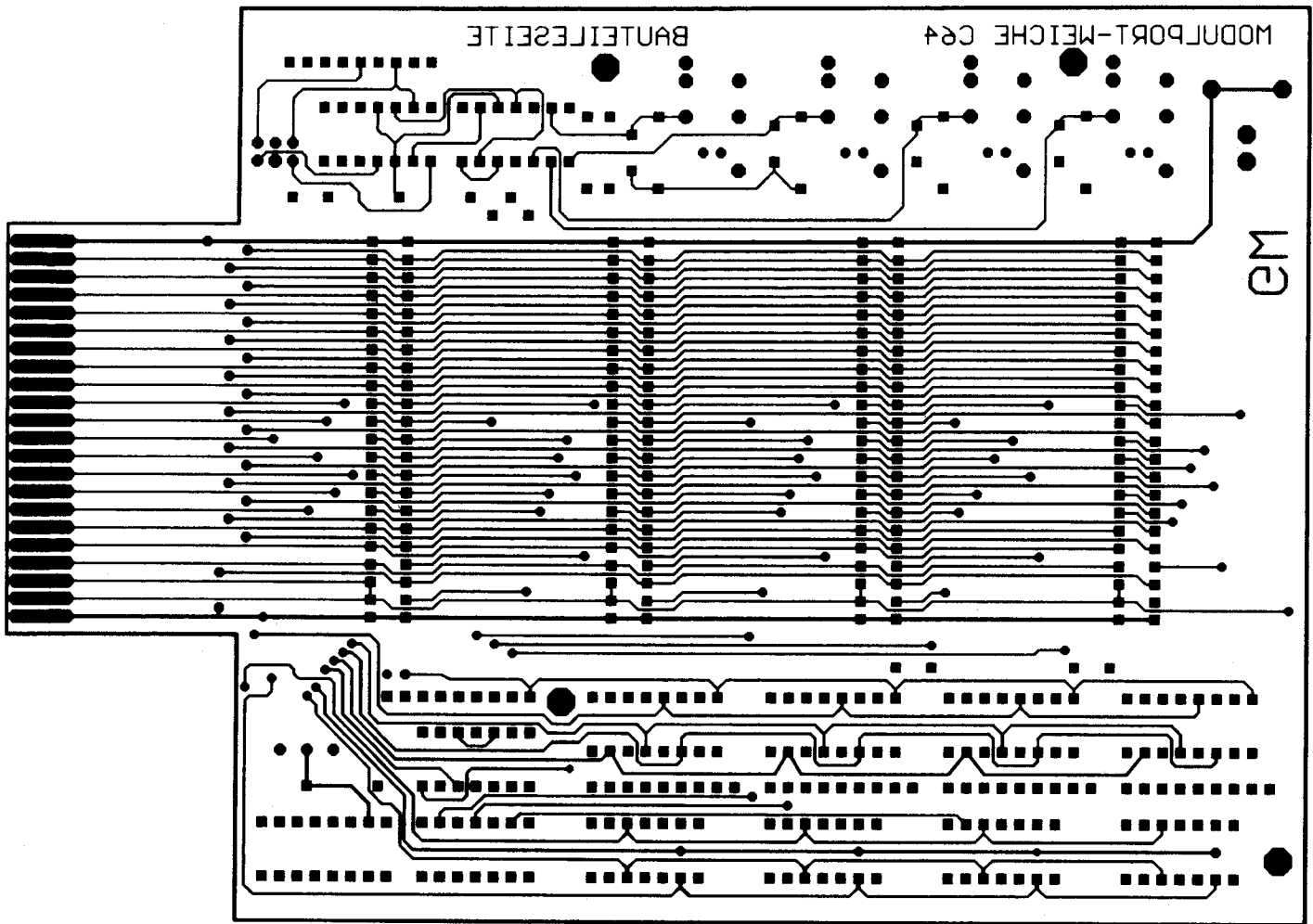
1 Layout (Bestückungsseite) der 4fach-Expansion-Port-Weiche
