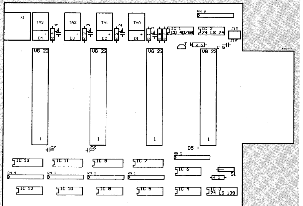
2 Bestückungsplan der 4fach-Expansion-Port-Weiche
