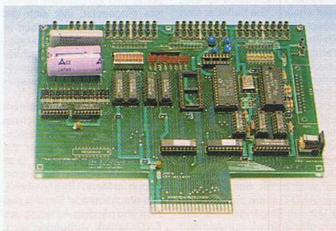
1 Mit dem Logik-Simulator lassen sich TTL-Schaltungen auf dem Computer entwickeln und testen
