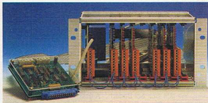
Das »VIS-System« wurde zur Regelung und Steuerung beliebiger Prozesse mit dem C64 entwickelt. Je nach Bedarf kann das System an die Bedürfnisse der Anwender angepaßt werden.
