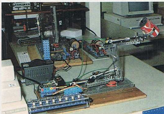
Bild 12. Ein durch den C 64 pneumatisch bewegter Roboterarm
