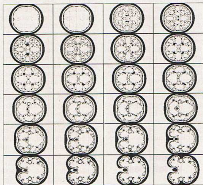
Bild 8. Magnetismus-Modelle imaginärer Stoffe in Abhängigkeit einer Materialkonstante
