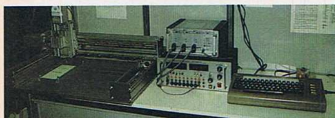
Bild 5. Ein professionell einsetzbares CNC-Frässystem für den C 64
