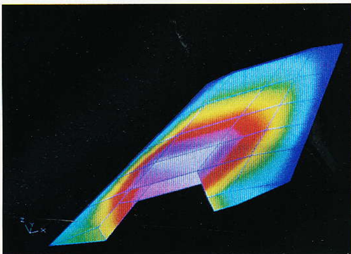
Bild 12. Je heller die Farbe, desto höher ist die Belastung des Tragflügels
