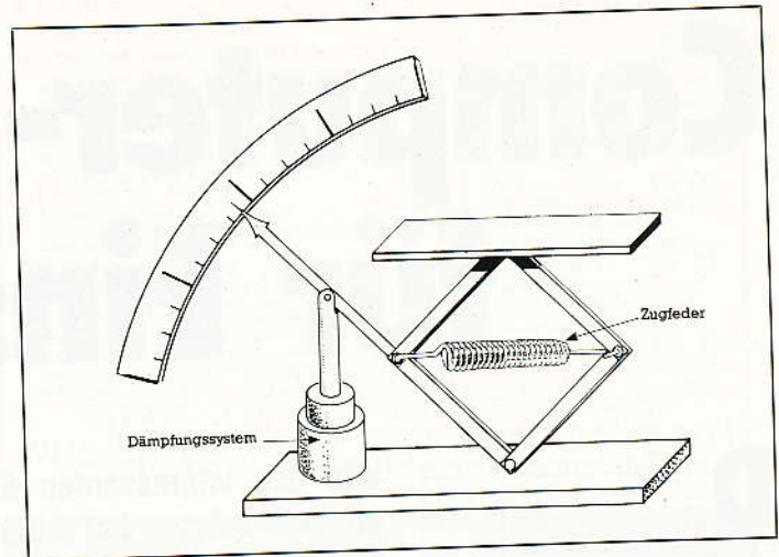
Bild 5. Aufbau einer Waage (schematisch)
