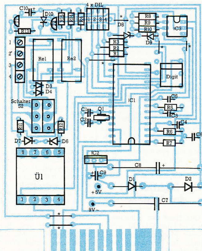
Bild 4. Bestückungsplan des Modems (* = Drahtbrücke)
