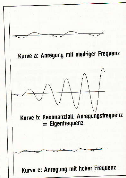
Bild 8. Erzwungene Schwingung
