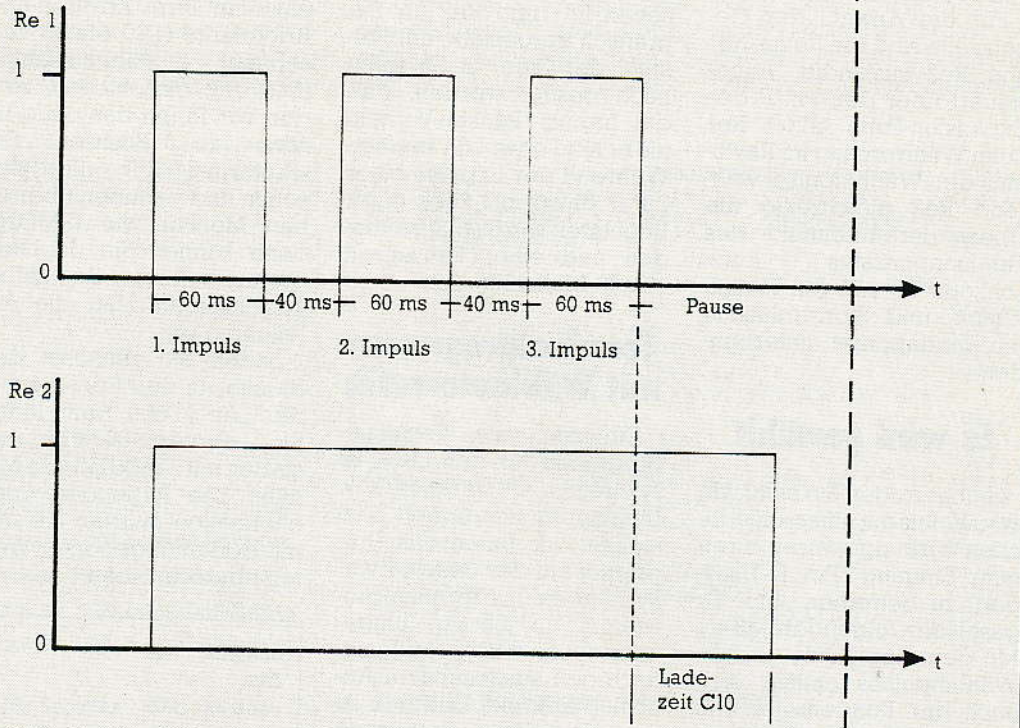
Bild 2. Die Signale der Relais Re1 und Re2 beim Wählen der Ziffer 3
