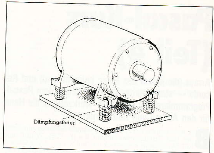
Bild 7. Motor auf Federdämpfung
