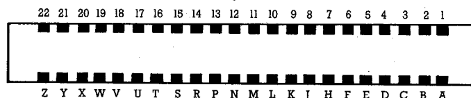
Der Expansion-Port des C 64 — von hinten gesehen
