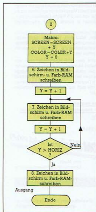
Bild 4. Flußdiagramm zum Programm RAHMEN
