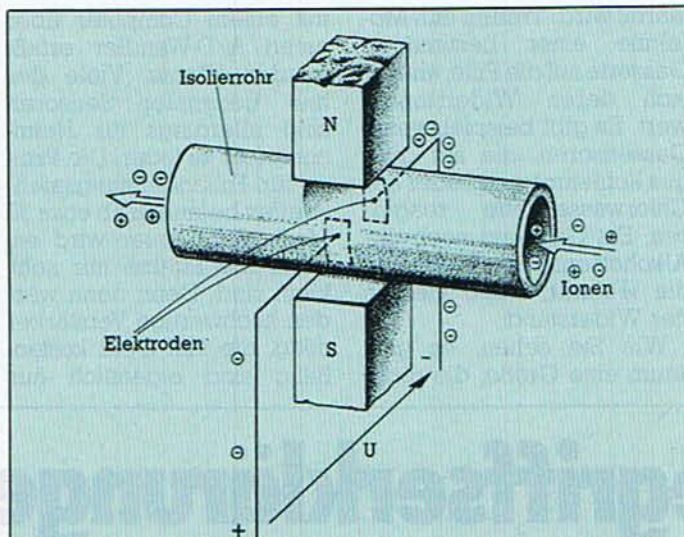
Bild 9. Eine besondere Art, Durchflußmengen zu messen, nutzt das Induktionsgesetz aus
