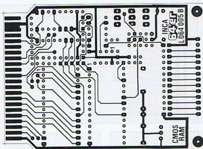
Bild 7. Layout der Platineoberseite
