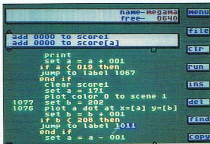
Bild 5. GameMaker — Programmieren mit dem Joystick
