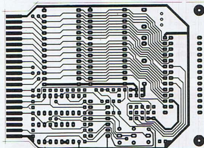
Bild 8. Layout der Platineunterseite
