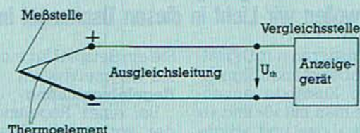
Bild 12. An den beiden Enden eines Thermoelementes kann man eine Spannung messen, die von der Temperatur abhängt
