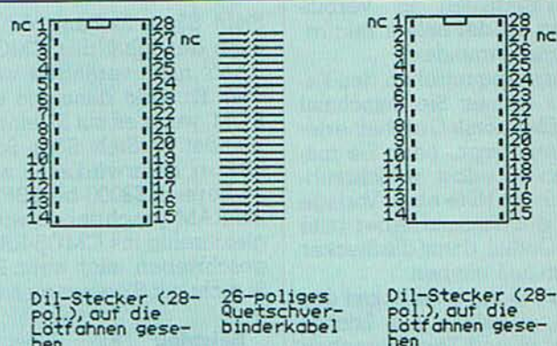
Bild 11. Verdrahtungsplan des Flachbandkabels
