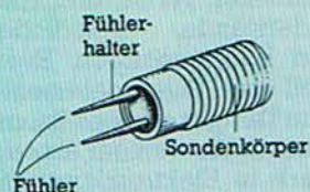
Bild 8. Die Hitzdrahtsonde dient zur Messung von Strömungsgeschwindigkeiten, aus denen leicht eine Durchflußmenge ermittelt werden kann
