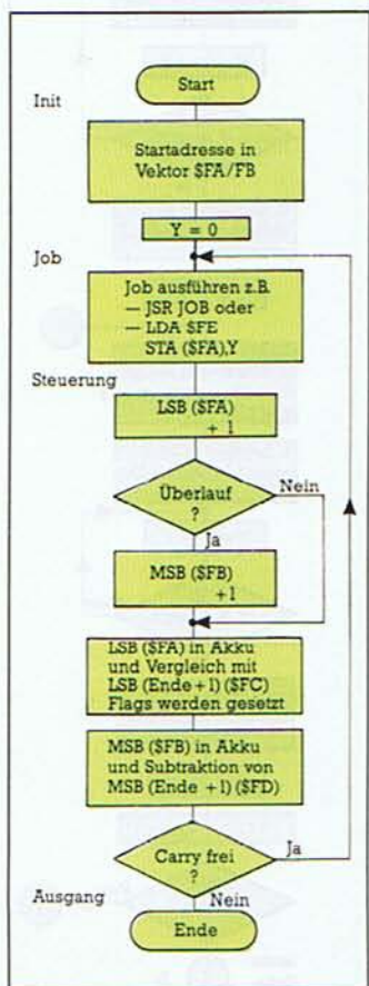
Bild 1. Flußdiagramm einer Doppelschleife für beliebige Laufzahlen
