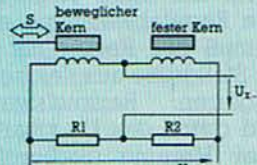
Bild 11. Schaltbild des Tauchankersensors
