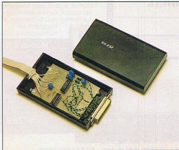
Bild 1. So kann das fertige Interface in einem Gehäuse aussehen
