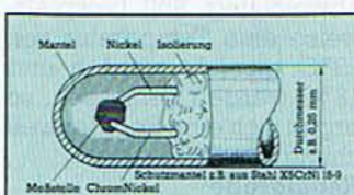
Bild 13. Thermoelemente werden normalerweise in ein Gehäuse eingebaut
