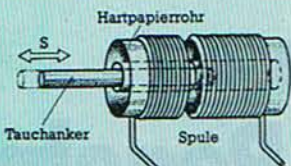
Bild 10. Der Tauchankersensor hat einen variablen Eisenkern. Ist der Eisenkern aus der Spule gezogen, ist die Induktivität nur gering. Befindet sich der Rundstab völlig in der Spule, ist die Induktivität groß.
