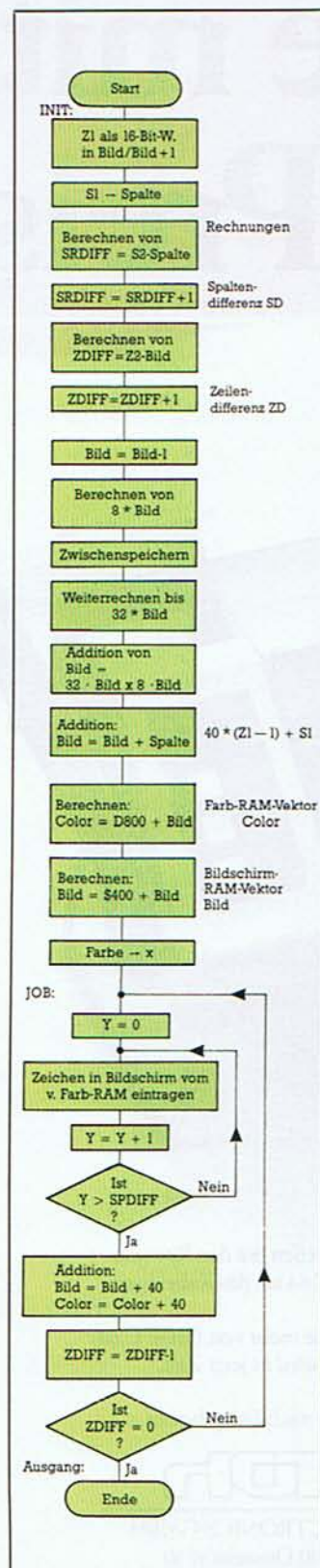
Bild 7. Flußdiagramm zum Programm »Teilbereich«
