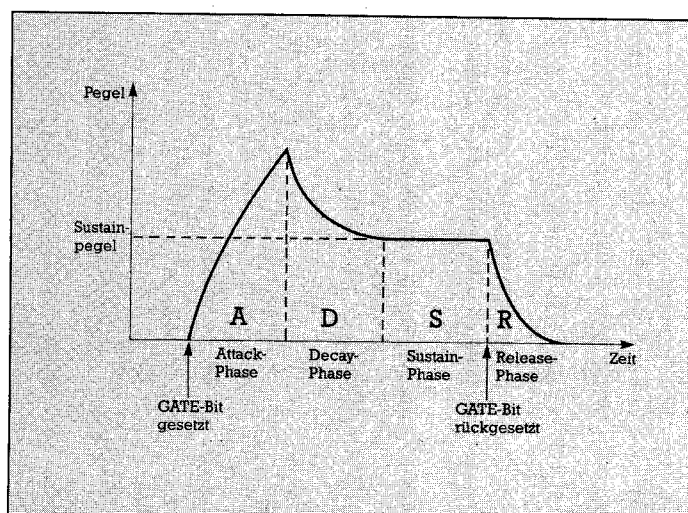
Bild 1. Der Verlauf von ADSR-Hüllkurven
