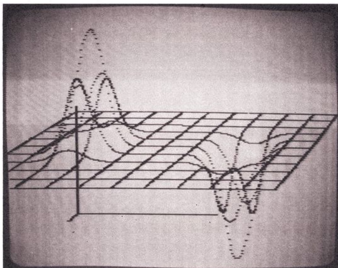
Bild 1. Die Funktion z = 5 + 5 \left( \sin \frac{\pi}{10} x \sin \frac{2\pi}{20} y \right)^{11} mit Ausgangspunkt (50,20,20) in Gitternetz-Darstellung
