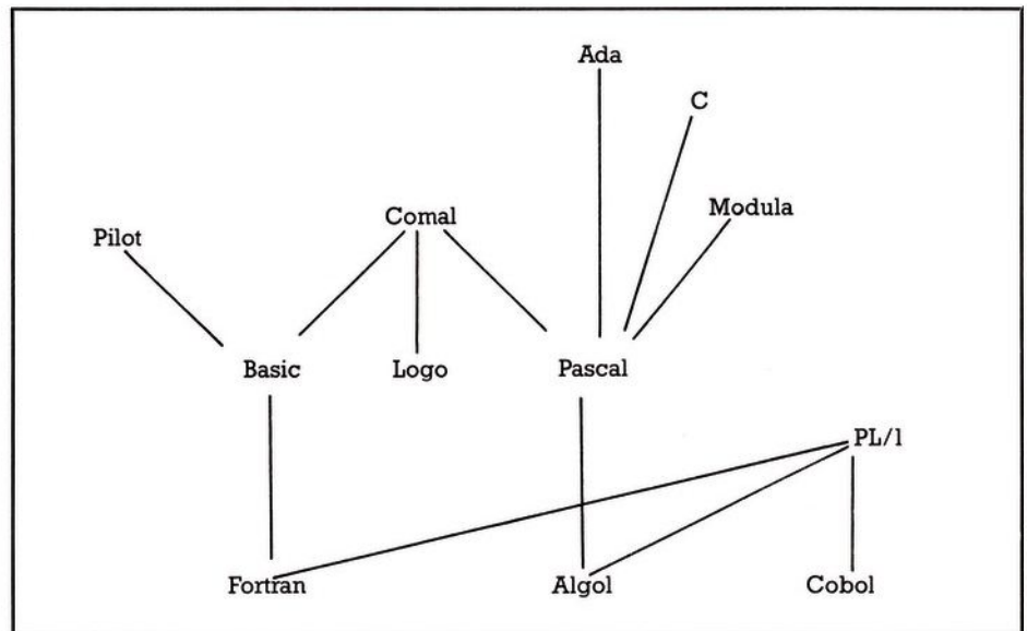
Der »Stammbaum« der höheren Programmiersprachen
