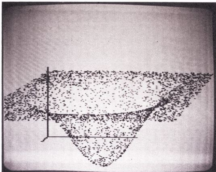
Bild 2. Die Funktion z = 5 - 5 \left( \sin \frac{\pi}{10} x \sin \frac{\pi}{10} y \right)^4 mit Ausgangspunkt (50,20,20) in der Darstellung mit zufällig ausgewählten Punkten
