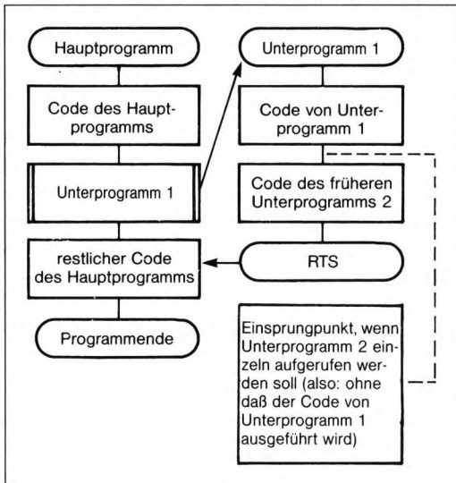
Bild 10.2: Der optimierte Algorithmus zur Verschachtelung von Unterprogrammen
