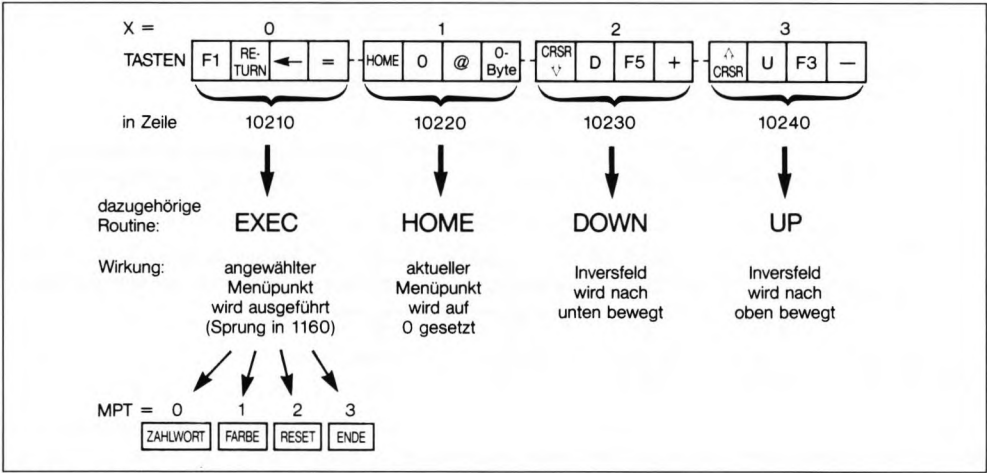
Bild 10.6: Die Tastaturabfrage aus Listing 10.11
