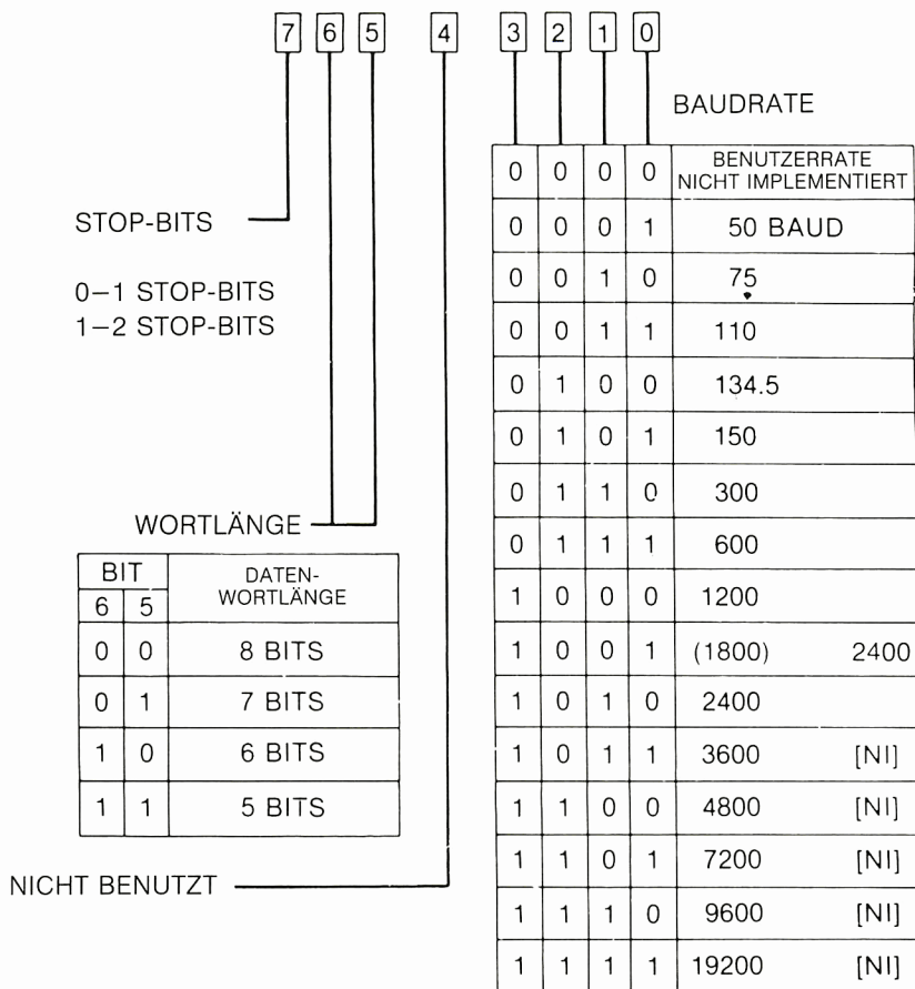
Abb. 6.1. Steuerregisterbelegung
