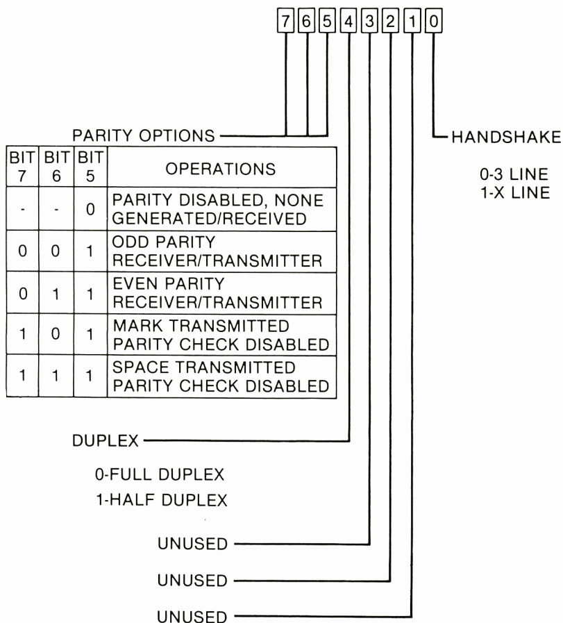
Abb. 6.2. Befehlsregisterbelegung
